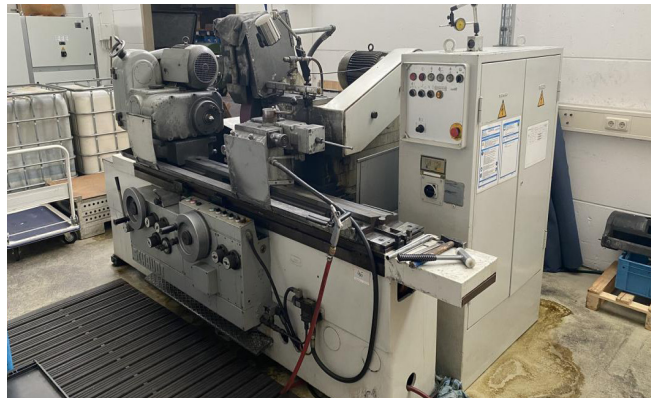
Pos. 46 1 Außenrundscheifmaschine SCHAUDT 511 N1000 1 External cylindrical grinding machine SCHAUDT 511 N1000
