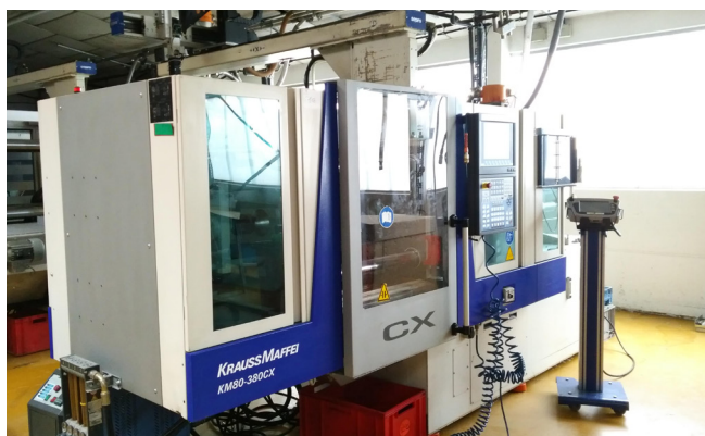
Pos. 116 1 Kunststoff-Spritzgießmaschine 1 Plastic injection moulding machine
