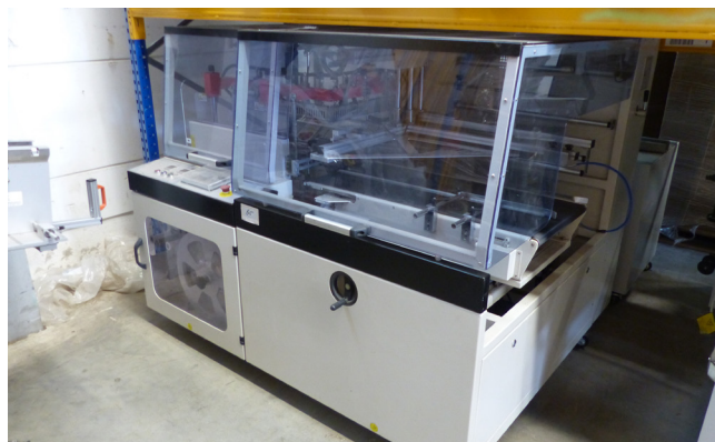
Pos. 65 1 autom. Schrumpffolienmaschine Amtec SPEEDshrink 40L 1 Shrink packaging machine Amtec SPEEDshrink 40L
