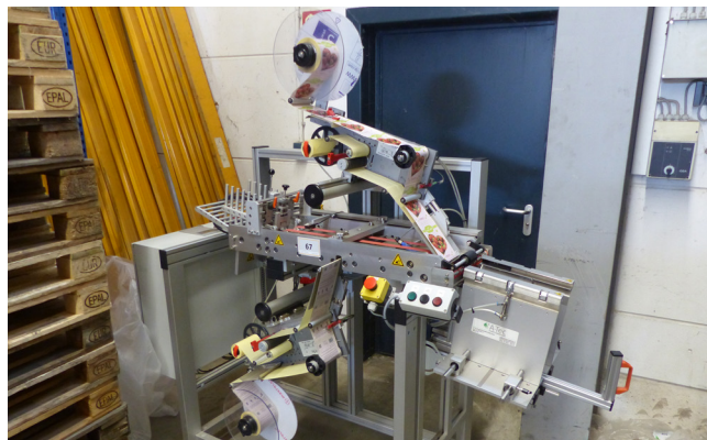
Pos. 67 1 Etikettieranlage A-TEC 1 Labelling system A-TEC
