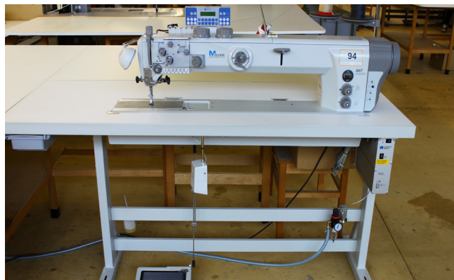
Pos. 94 1 Einnadel-Doppelstepstich-Langarm-Industrienähmaschine 1 Single-needle lockstitch long arm industrial sewing machine DÜRKOPP-ADLER
