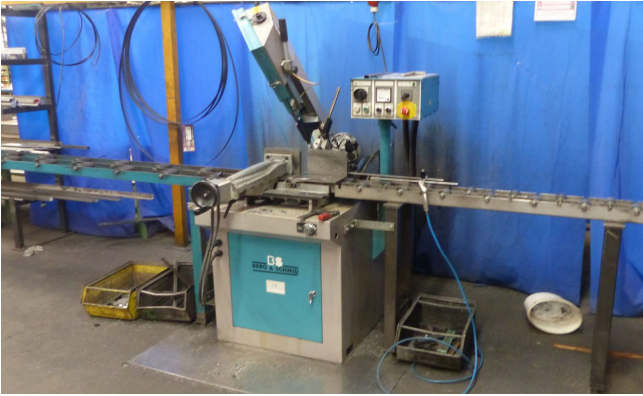
Pos. 59 1 Gehrungsbandsäge BERG & SCHMIDT GBS242 DG, Bj. 2014 1 Mitre band saw BERG & SCHMIDT GBS242 DG, YOM 2014
